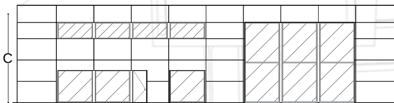
FACHADA LATERAL
