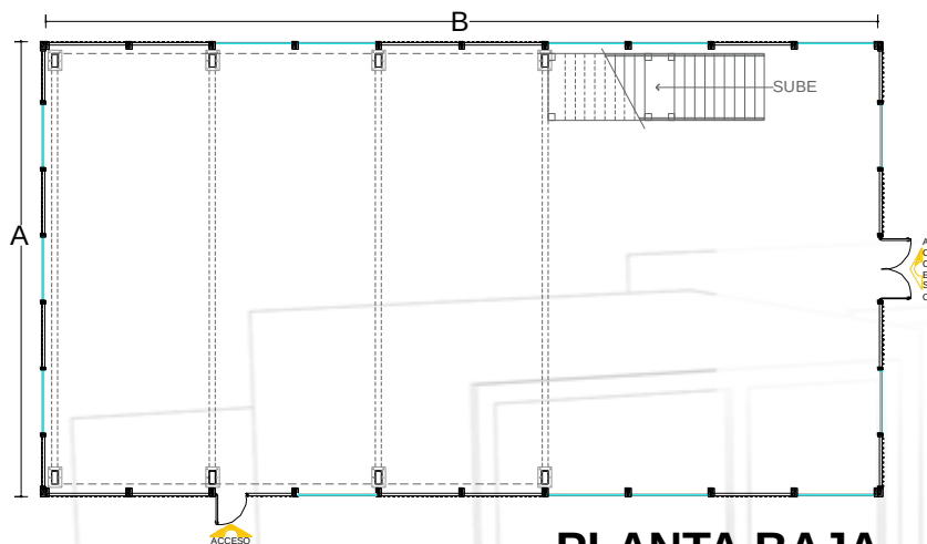
PLANTA BAJA
