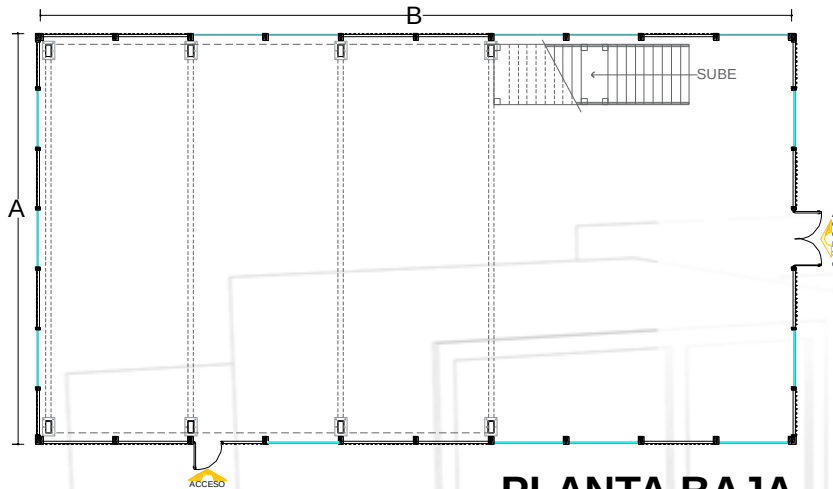
PLANTA BAJA
